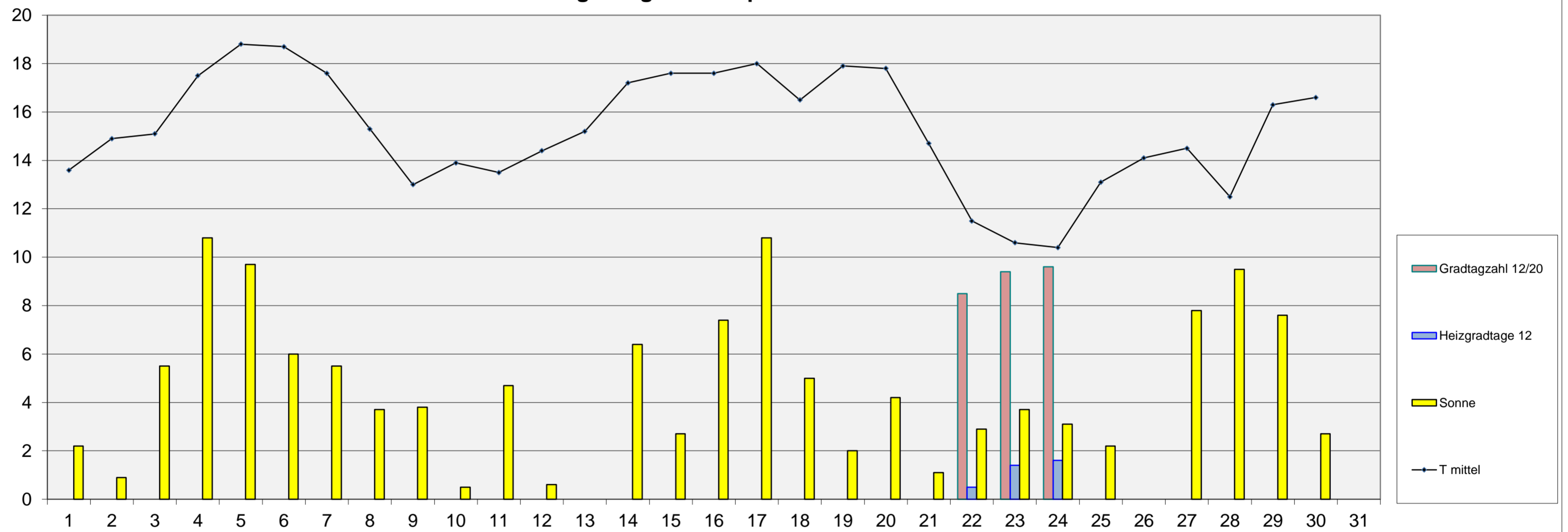
Energiediagramm September 2014
